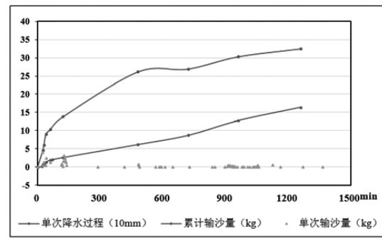
图5 输沙量在单次降水过程的变化情况
