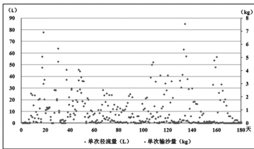
图4 单次径流量和输沙量相关性图谱
