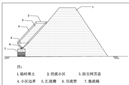
图 1 径流小区侧视图
