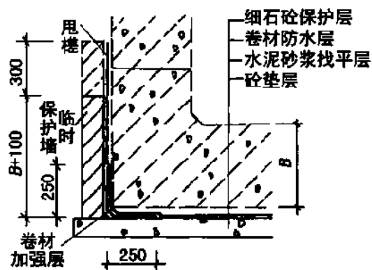
图1 防水施工示意图
