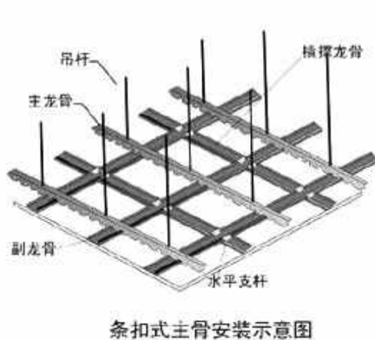
图2 龙骨安装方法示意图
