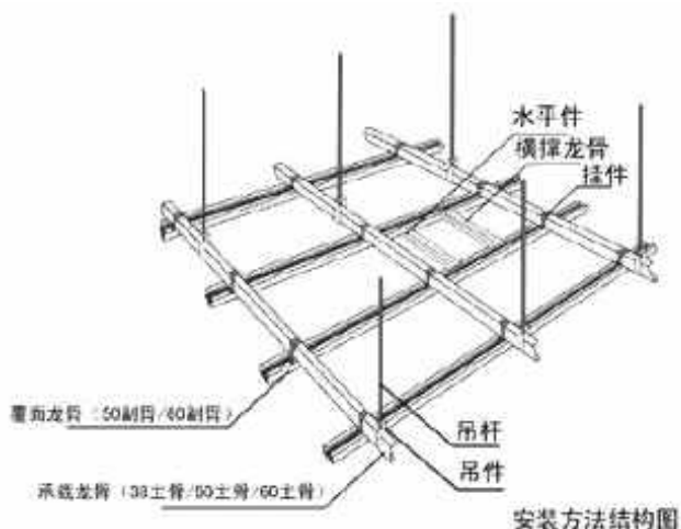
图2 龙骨安装方法示意图
