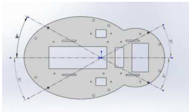
图 2.5 主体结构
