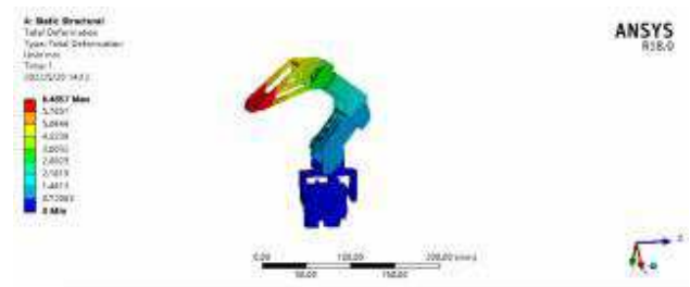
图 2.8 形变图
