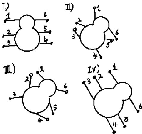
图 3.3 三足步态定点转弯规划图
