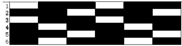
图 3.4 仿生机器人四足步态的腿部相位图
