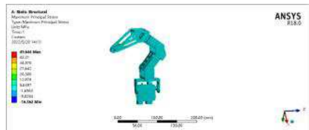
图 2.9 最大主应力图
