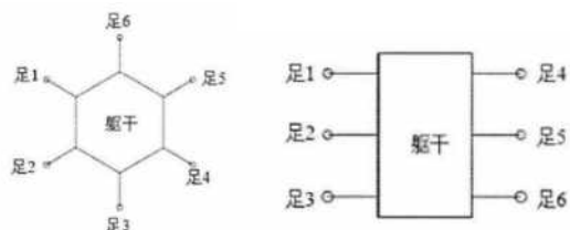
图 2.3 均匀式分布图 2.4 轴对称的分布
