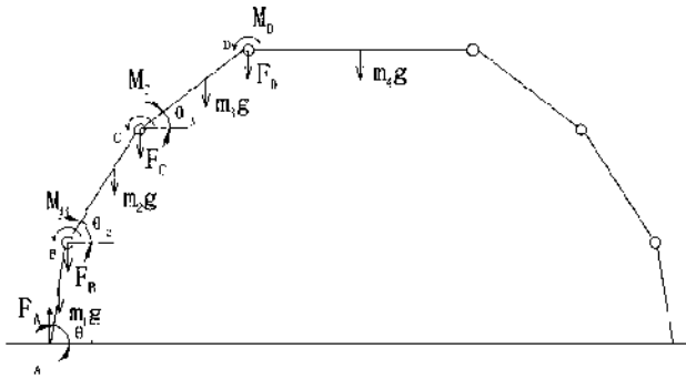
图 2.7 力学分析模型
