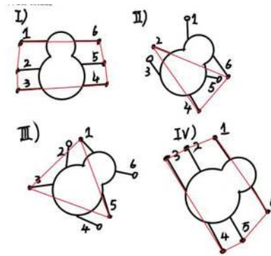
图 3.10-2 三足步态定点转弯
