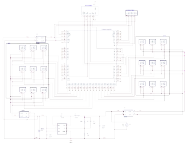
图 4.2 仿生蜘蛛机器人电路
