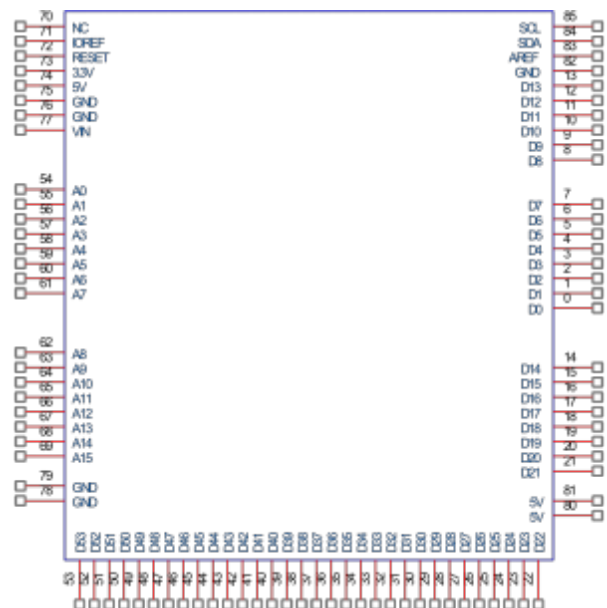
图 4.3 Arduinomega2560 引脚图
