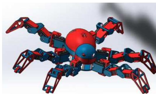
图 2.6 仿生蜘蛛机器人整体结构
