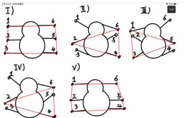
图 3.10-1 三足步态直线行走
