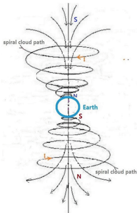
图1 位于地球两极的偶极磁场
