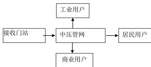
图1 输配系统流程图
