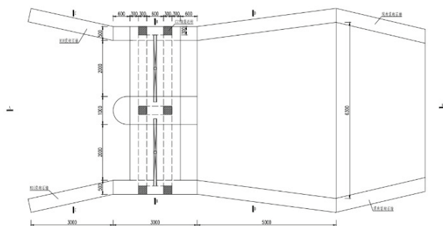
新屋闸平面图
